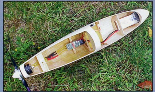
Le fuselage aménagé avec la motorisation.
