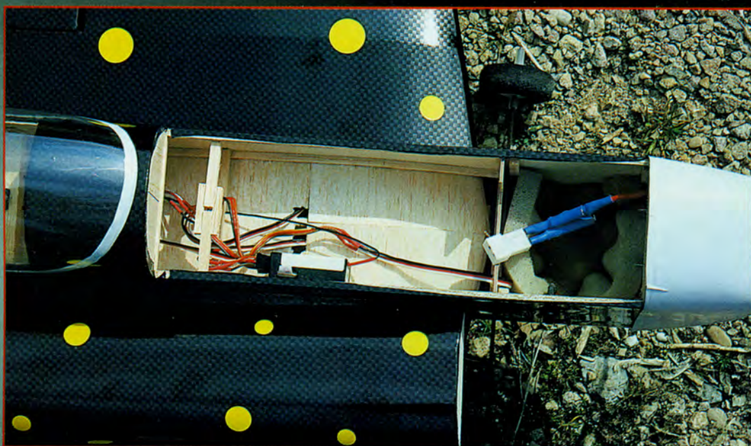
Sous le capot amovible, le récepteur et le logement de l'accu. Le variateur a été installé dans le capot avant.
