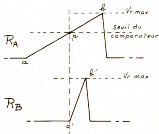
Fig. 4. – Les rampes A et B du double balayage.
